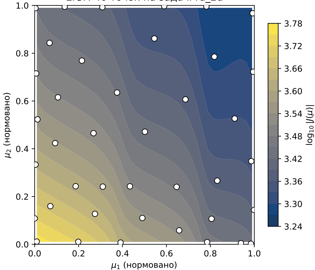
EIGF: 40 точок на задачі rd_2d
